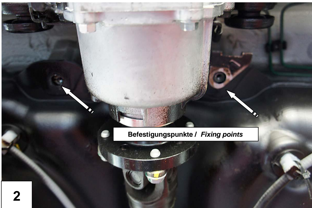
Befestigungspunkte Konsole "B" / Fixing points brac
