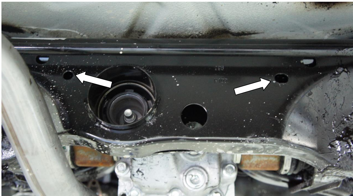
Befestigungspunkte Schutzplatte "C" / Fixing points skid plate "C"
